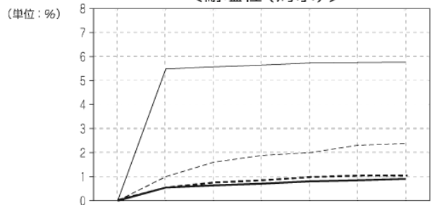
〔耐塩性(海水)〕
